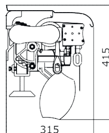
Homlokzati rögzítés védőfedővel
